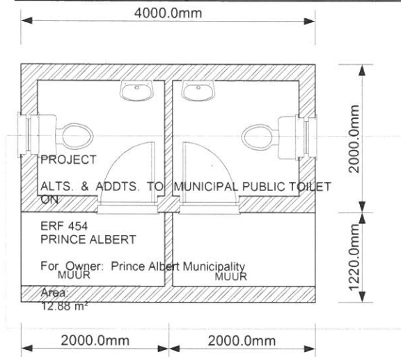
VLOERPLAN
