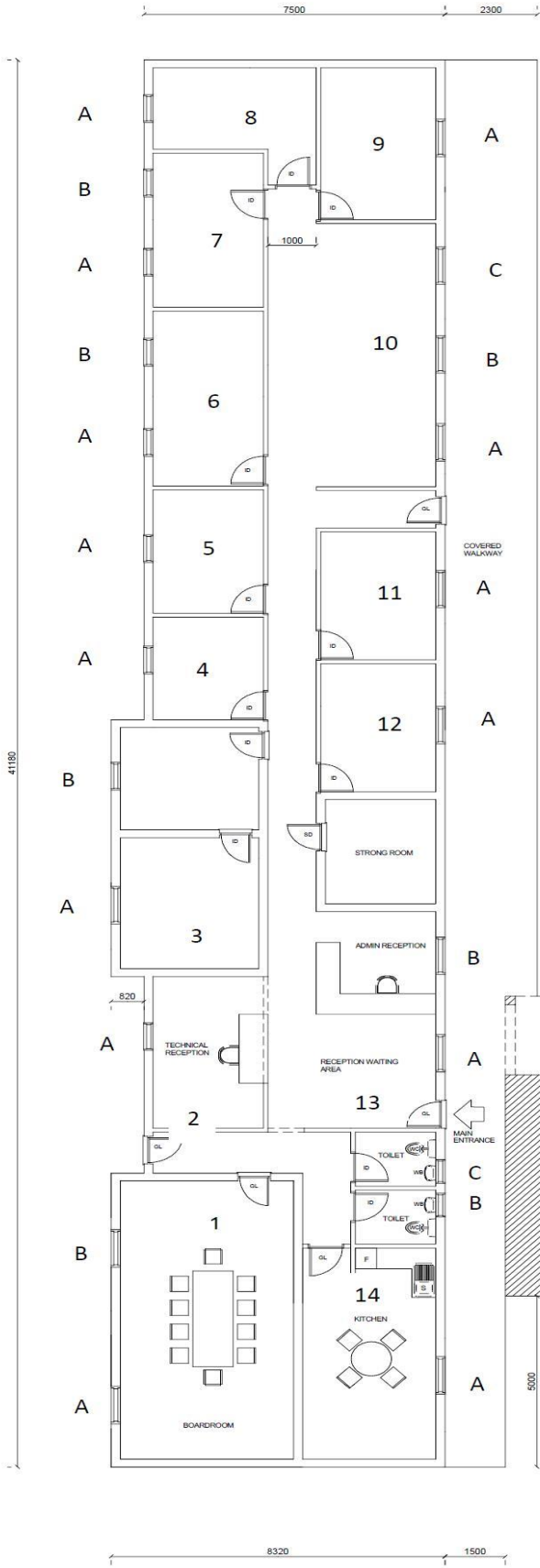
SITE PLAN 1:100
